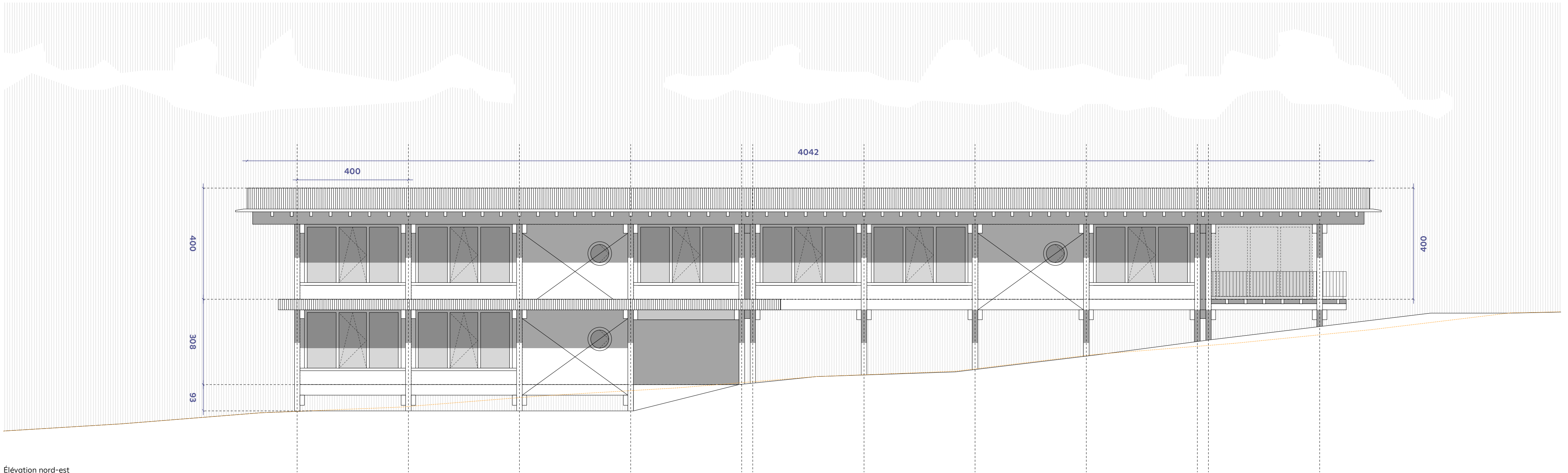
Élévation nord-est
